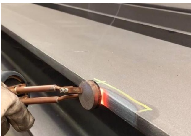
Materiál se přehřeje jen na požadovaných místech.
