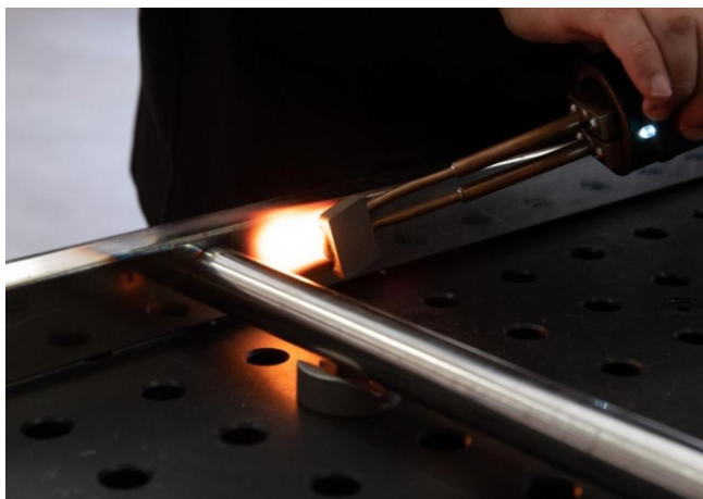
Může sloužit pro rovnání svařenců po svařování.
